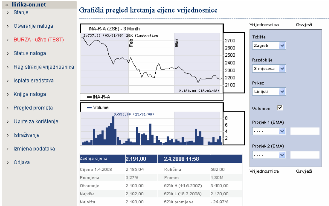
Slika 14. Grafički pregled kretanja cijene vrijednosnica
